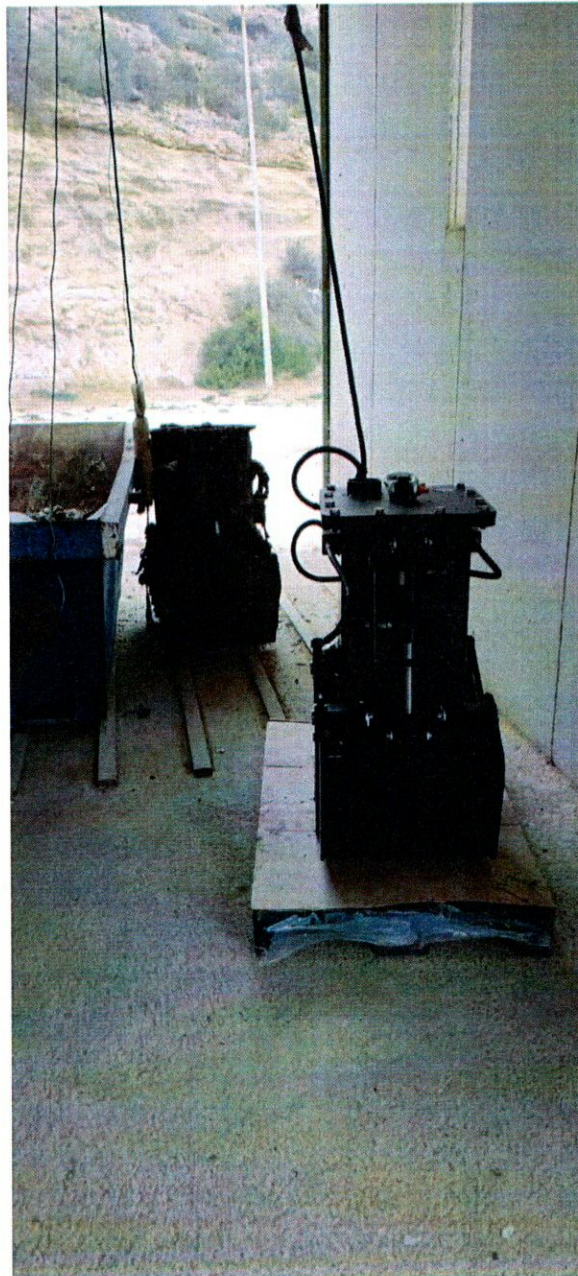
Fotografía de la izquierda con la cuchara bivalva nueva y de la derecha con la cuchara antigua inservible ya desconectada y la nueva ya instalada y en funcionamiento
