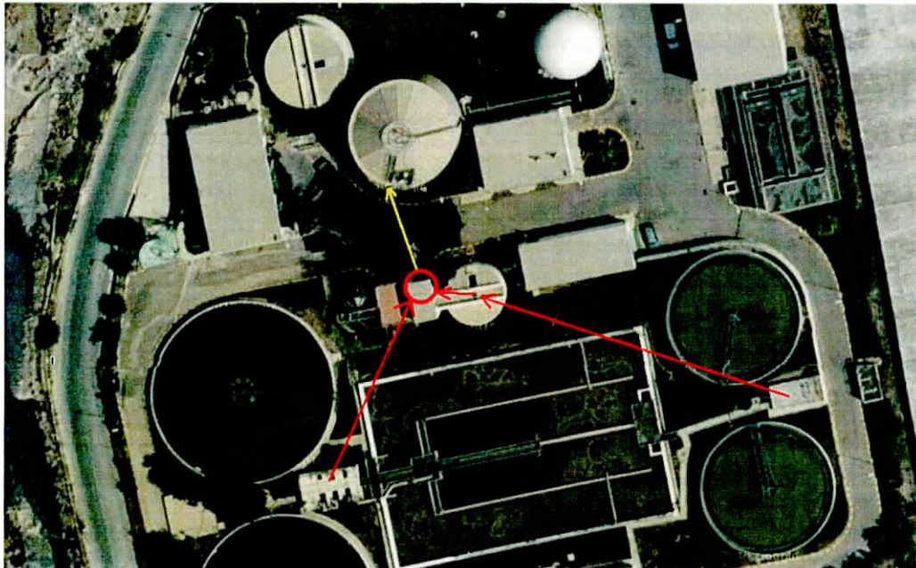
Fotografía aérea de la EDAR El Ejido, con las líneas de fangos primarios y secundarios en rojo, que terminan en la cámara de fangos mixtos, desde donde se bombearían al digester según la flecha en amarillo
