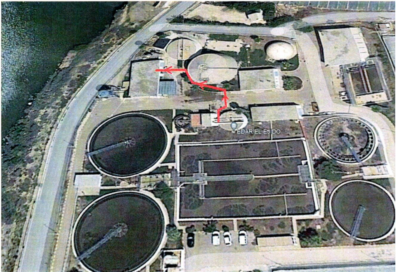
Fotografía de la conducción temporal en superficie instalada para conectar la salida del espesador con la alimentación de las bombas de deshidratación, haciendo by-pass del depósito de almacenamiento de fangos tampón
