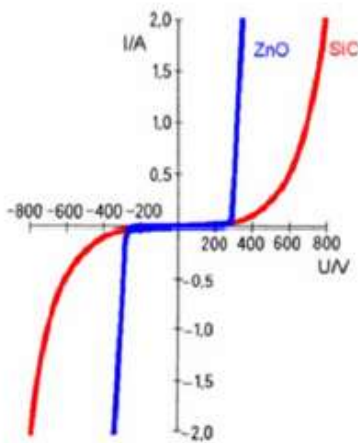
Curva de funcionamiento de un varistor
