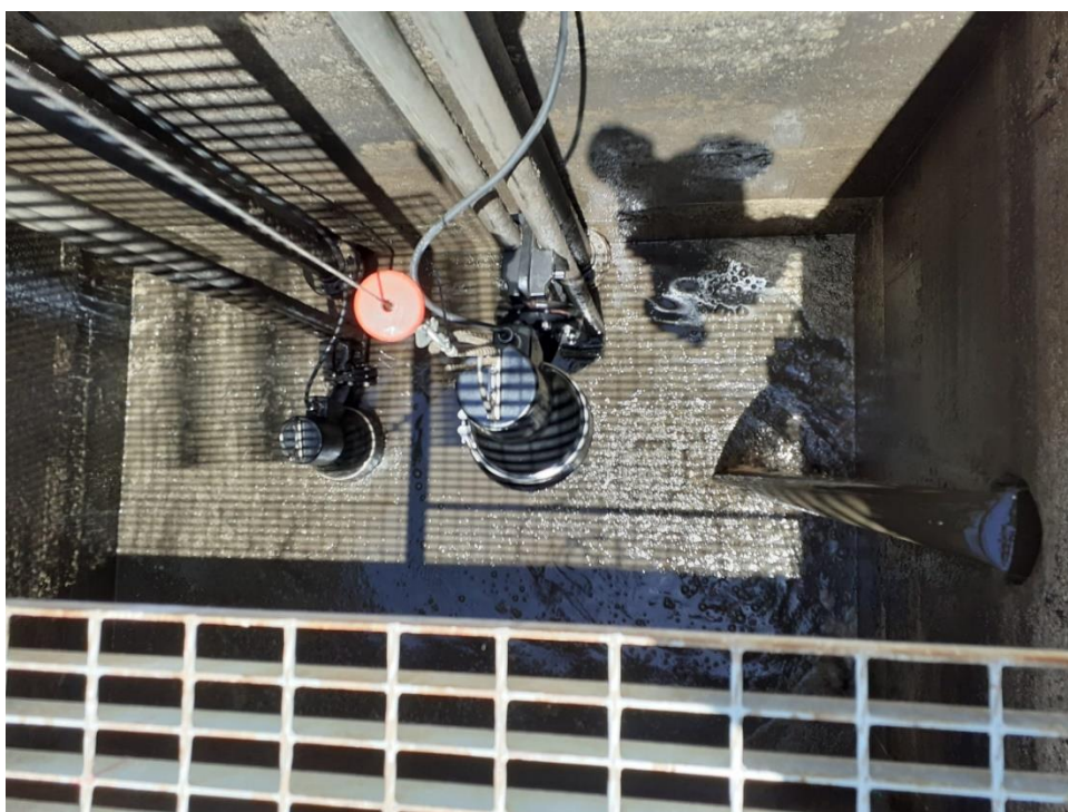
Bombas instaladas en el bombeo de vaciados de la EDAR Adra
