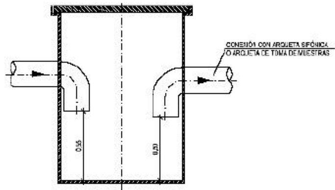
ALZADO SECCIÓN
