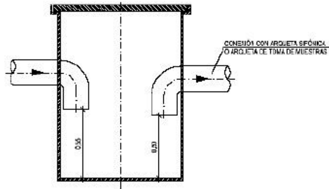
ALZADO SECCIÓN
