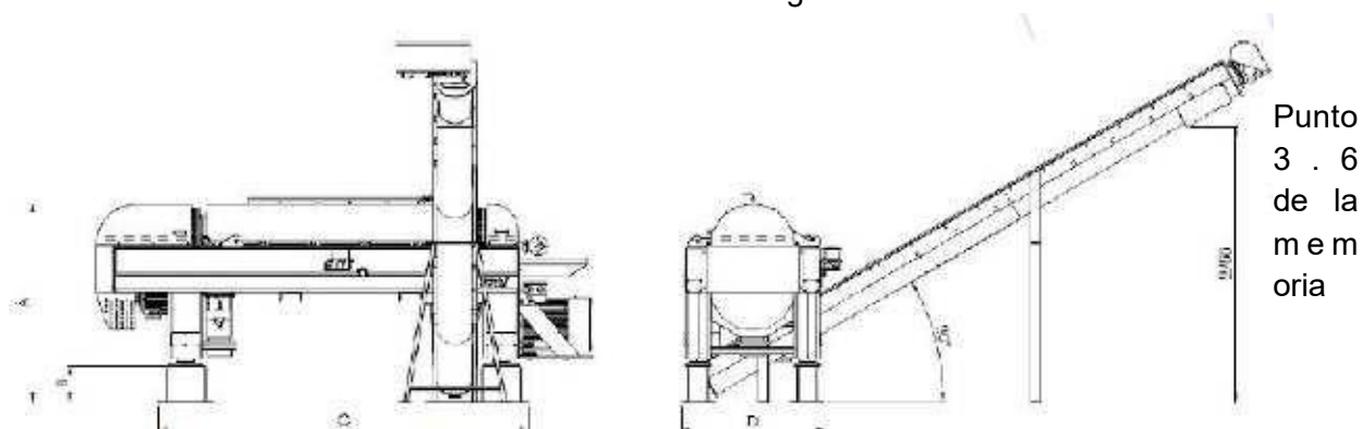
Figura 14. Dimensiones decanter
