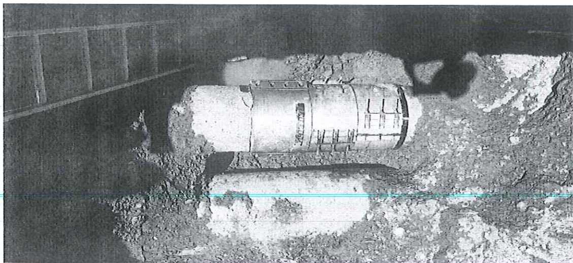
Conducción de impulsión de la EBAR Géminis a la EDAR Adra de FD400 con las 3 abrazaderas de reparación instaladas
