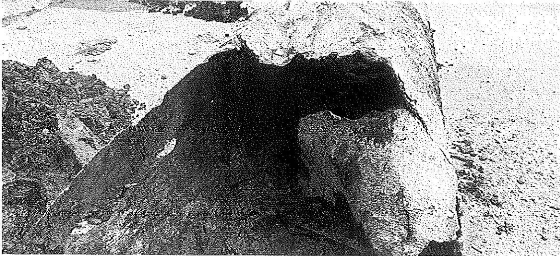
Estado de desintegración de la conducción de FD400 extraída
