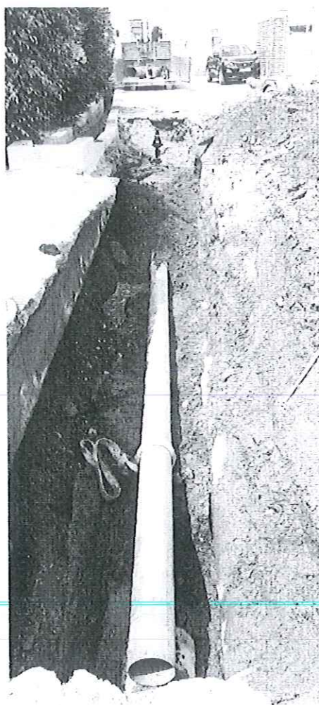
Tubos de PVC DN250 instalados con ventosa sustituyendo los de FD DN400 hasta conectar con tramo original
