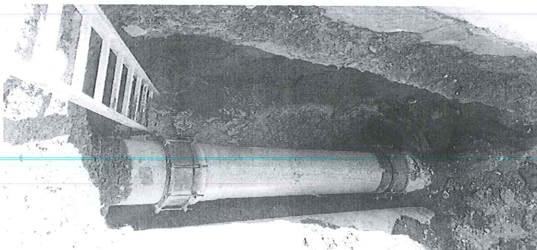
Tramo de conducción sustituida y nueva fuga detectada
