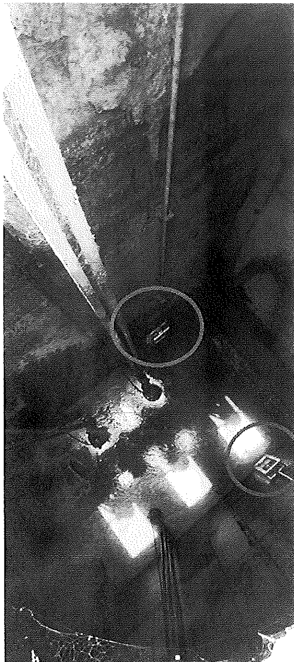
Vista de ambas compuertas de recirculación instaladas desde la arqueta de recirculación
