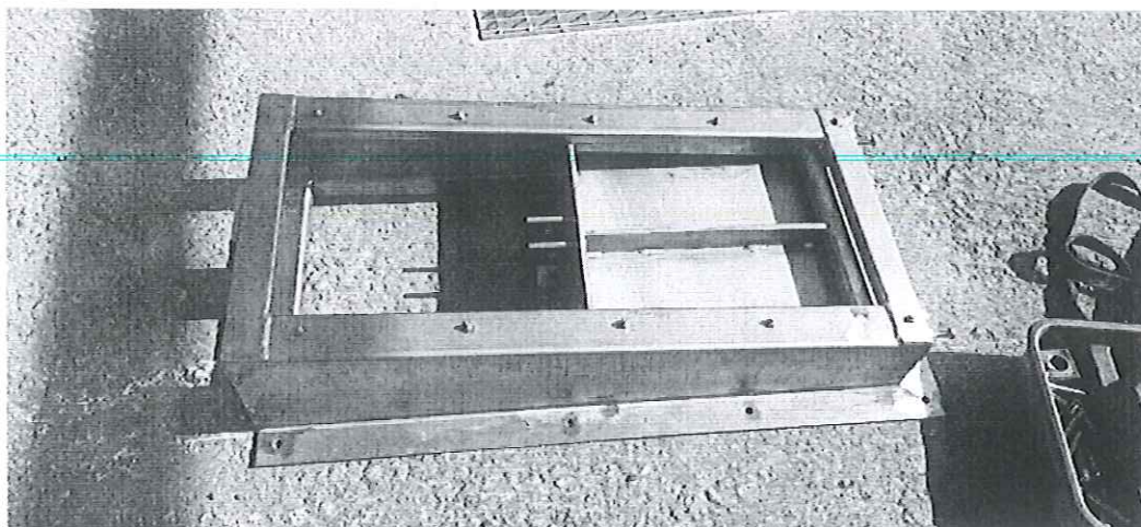
Compuerta de decantador secundario B hacia recirculación desinstalada y la nueva que se ha instalado
