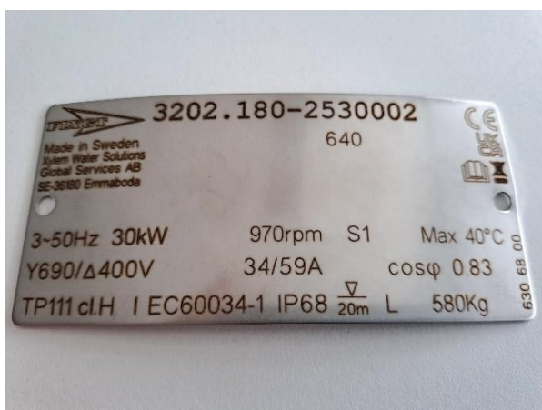
Detalle placa bomba reserva EBAR Paraíso del Mar
